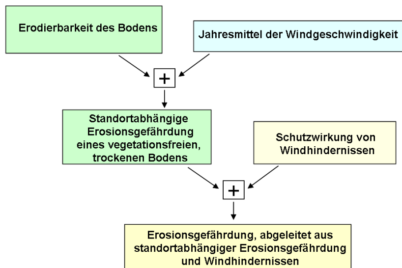
Abb. 1: Vorgehensweise bei der Ermittlung der Erosionsgefährdung durch Wind (nach DIN 19706, verändert)
