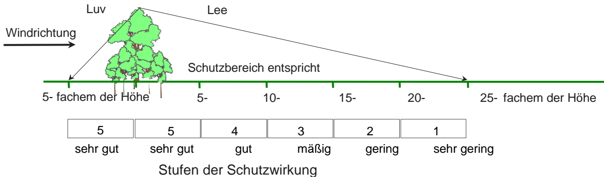
Abb. 2: Stufen der Schutzwirkung und Einteilung von Schutzbereichen vor und hinter Windhindernissen (aus DIN 19706)
