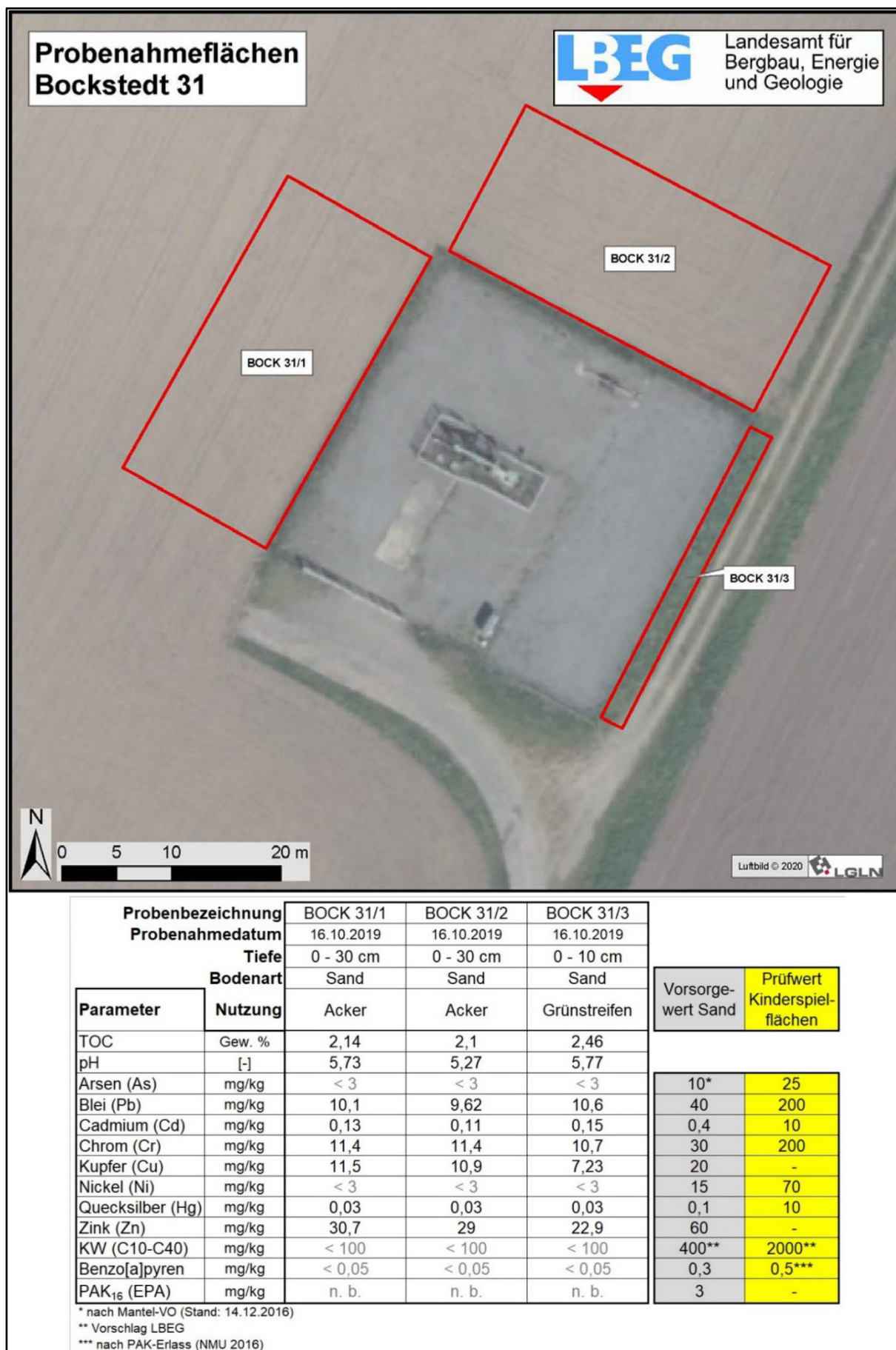
Abb. 3: Untersuchungsstandorte und Analyseergebnisse Bockstedt 31
