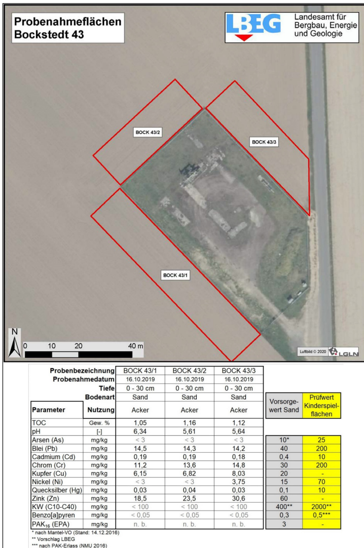
Abb. 5: Untersuchungsstandorte und Analyseergebnisse Bockstedt 43
