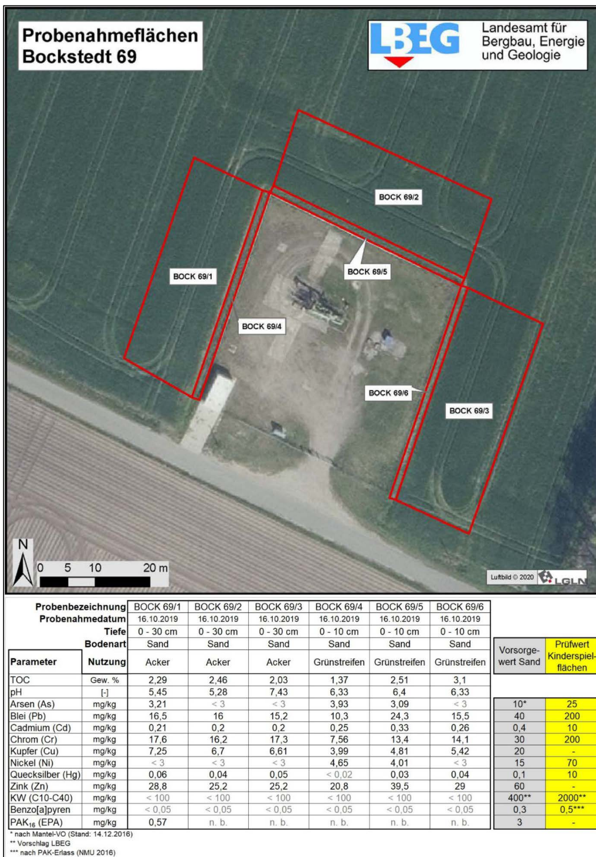
Abb. 6: Untersuchungsstandorte und Analyseergebnisse Bockstedt 69
