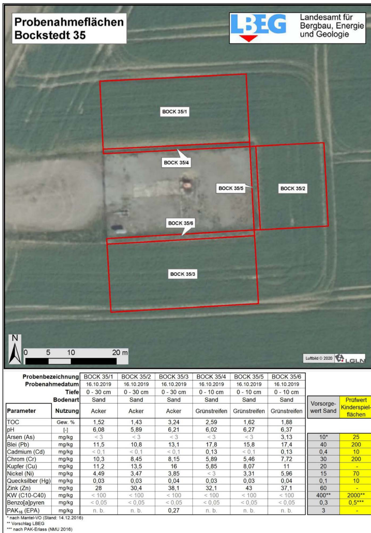
Abb. 4: Untersuchungsstandorte und Analyseergebnisse Bockstedt 35
