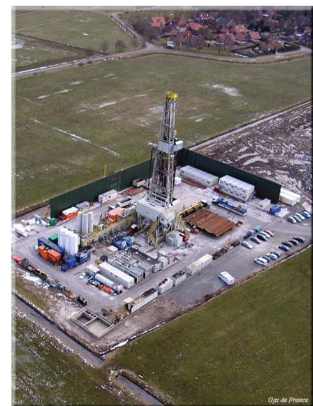
Tiefbohranlage (Lokation Gasfeld Leer)
