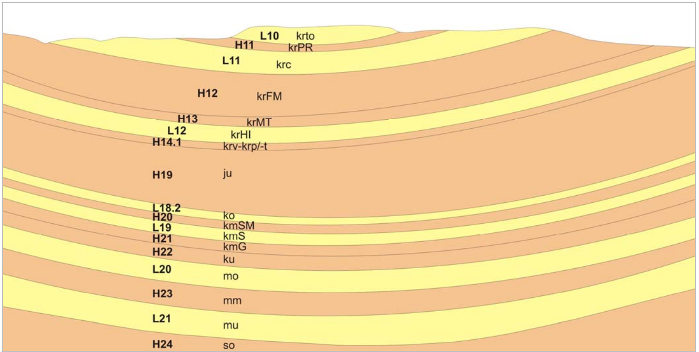
Abb. 3: Schematischer hydrogeologischer Schnitt, Festgestein, Südniedersachsen, Mesozoikum, ungestört.
