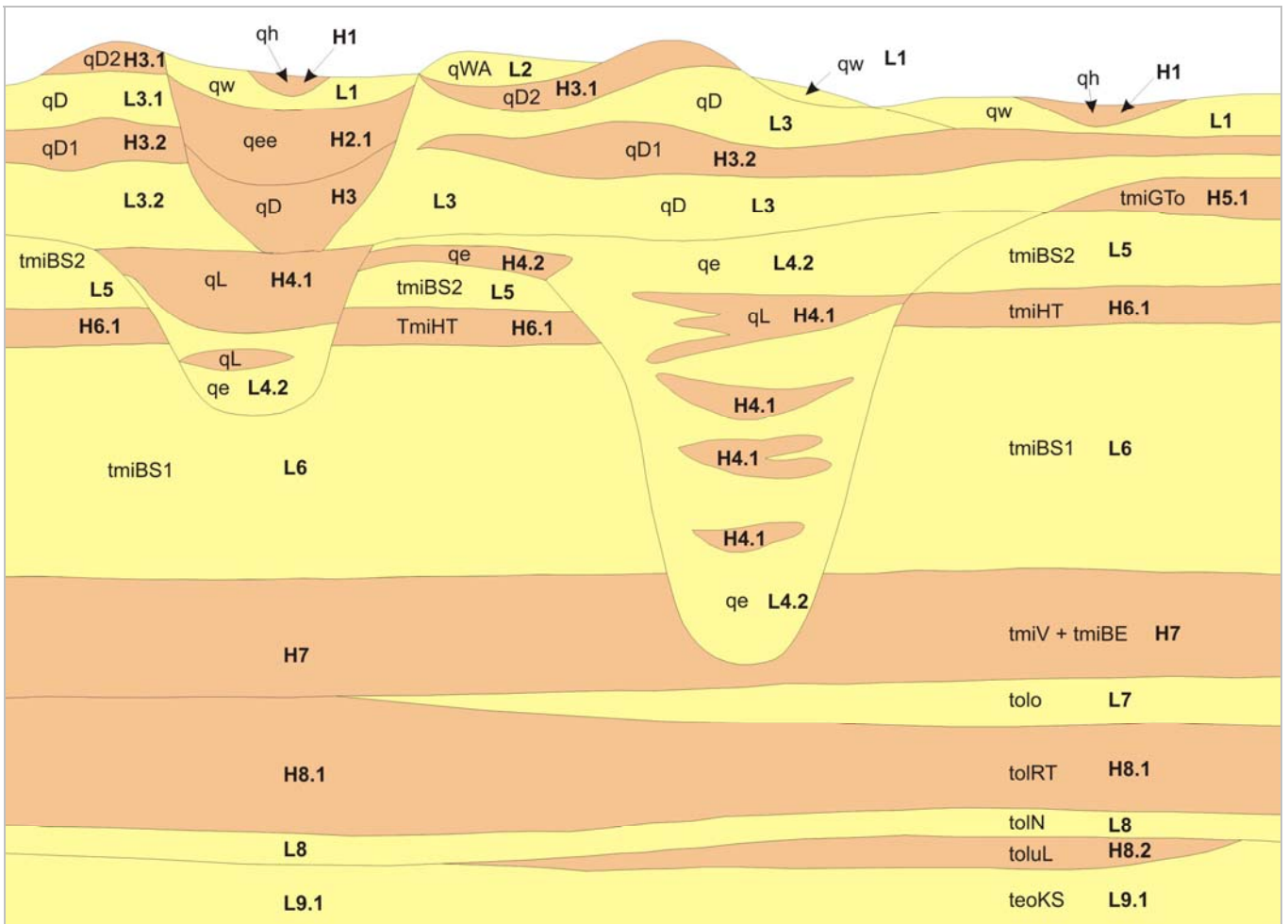
Abb. 2: Schematischer hydrogeologischer Schnitt, Lockergestein, Nordostniedersachsen, Känozoikum.
