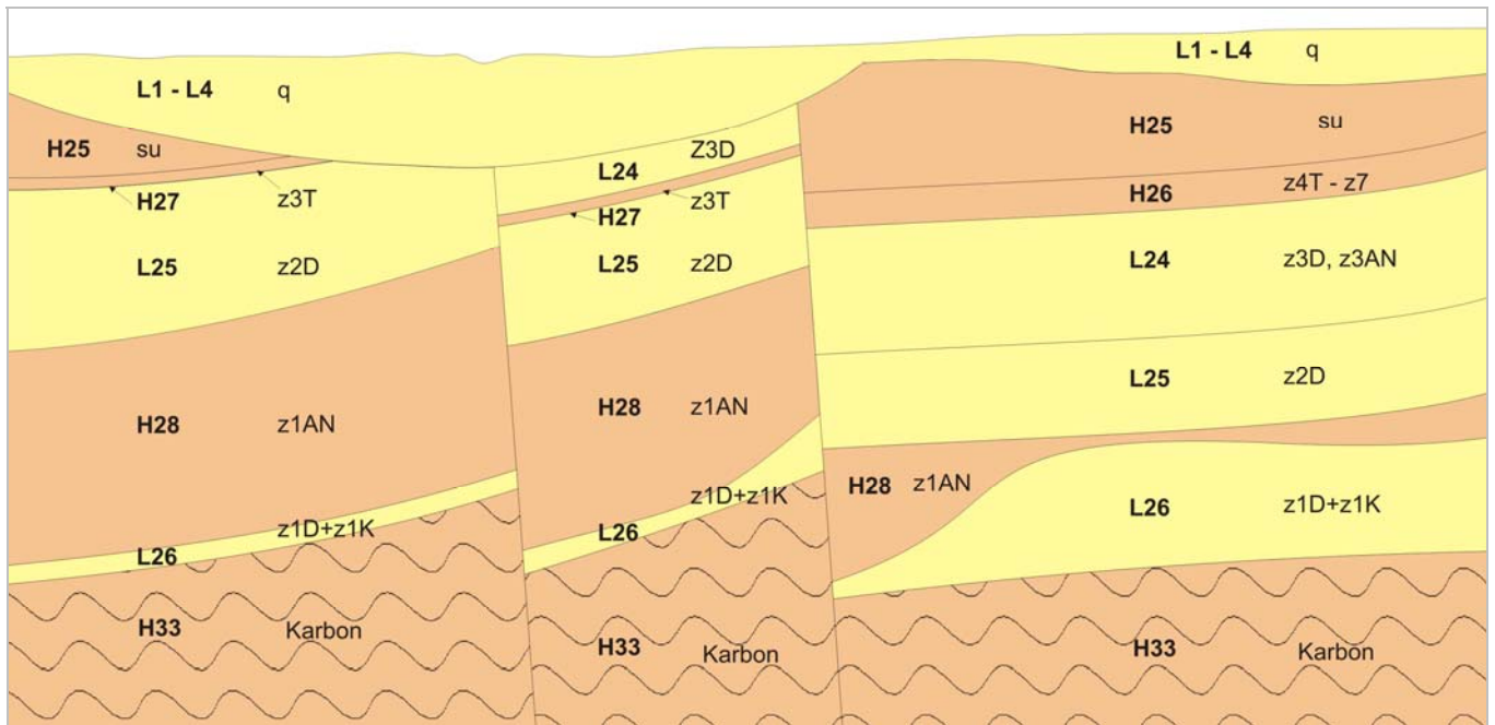
Abb. 5: Schematischer hydrogeologischer Schnitt, Festgestein, Südniedersachsen, Paläozoikum, Südharz.
