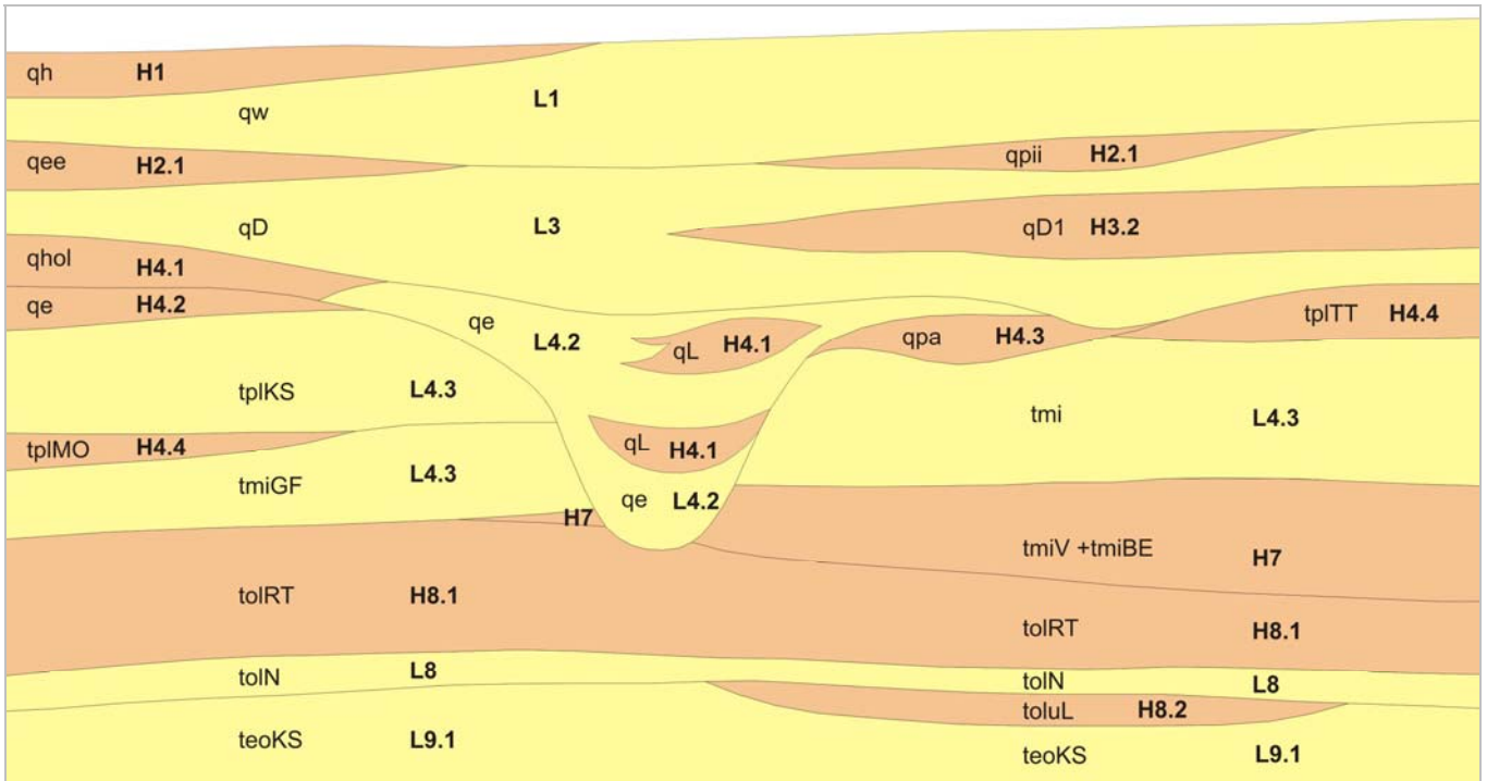
Abb. 1: Schematischer hydrogeologischer Schnitt, Lockergestein, Nordwestniedersachsen, Känozoikum.
