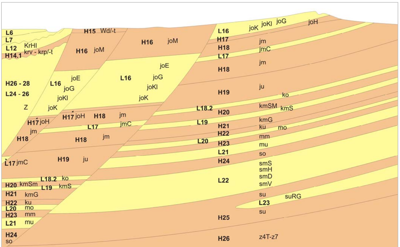
Abb. 4: Schematischer hydrogeologischer Schnitt, Festgestein, Südniedersachsen, Mesozoikum, gestört.
